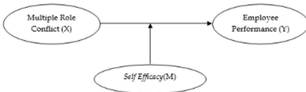
Gambar 1. Kerangka Penelitian
